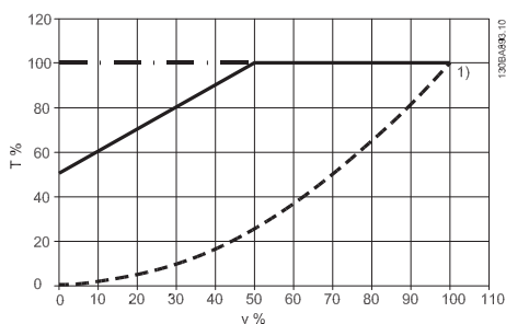
Максимальная нагрузка для типового двигателя при температуре 40 °C с приводом AF-600 FP от преобразователя частоты типа VLT FCxxx
