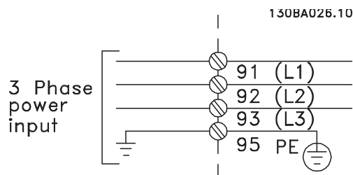
Рисунок 5.1: Клеммы сетевого питания и заземления.
