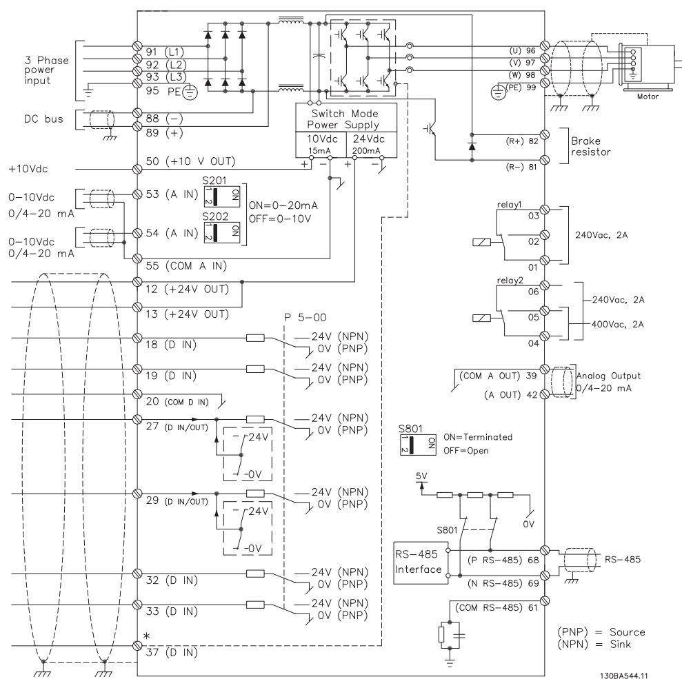
Рисунок 5.41: Схема электрических соединений всех клемм. (Клемма 37 предусмотрена только в блоках с функцией аварийного останова.)
