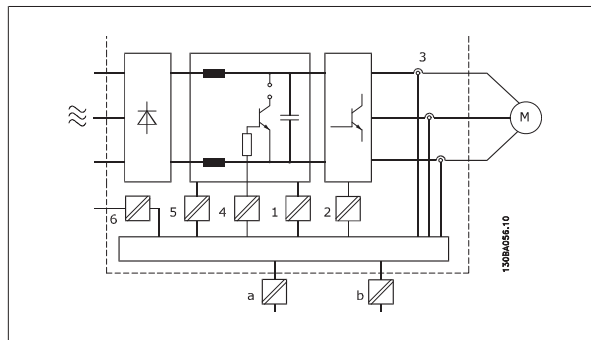
Рисунок 3.3: Гальваническая развязка
