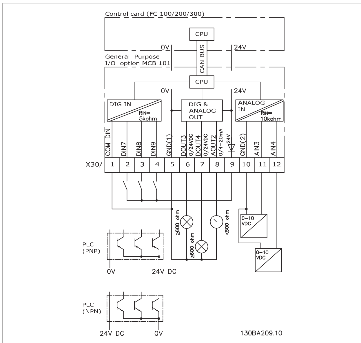
Рисунок 8.1: Принципиальная схема
