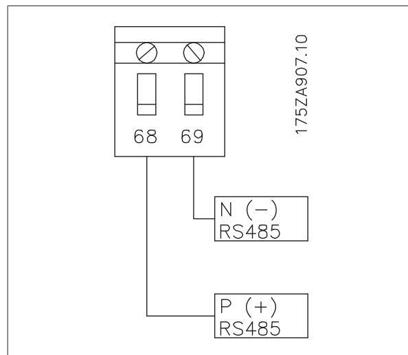
Рисунок 9.1: Подключение клемм сети
