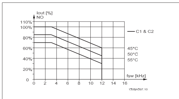
Рисунок 4.11: Снижение тока I_{out} для различных значений T_{AMB, MAX} в случае корпуса C при использовании модели коммутации 60 PWM в режиме нормального крутящего момента (перегрузка по крутящему моменту 110 %).
