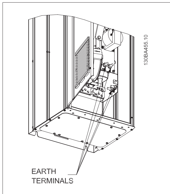
Рисунок 6.42: Расположение клемм заземления, IP21 (NEMA, тип 1) и IP54 (NEMA, тип 12).
