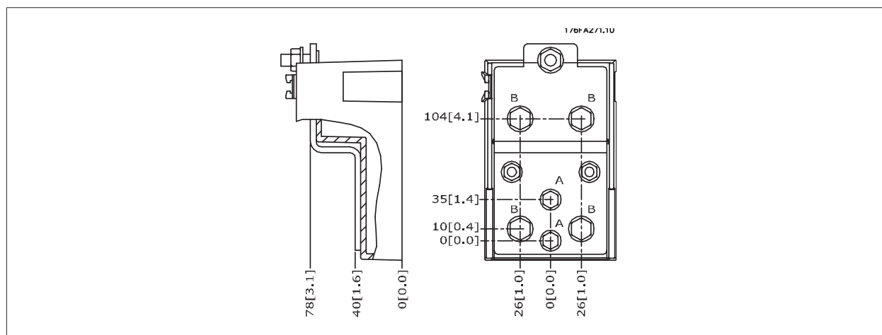
Рисунок 6.12: Конструкция клеммы
