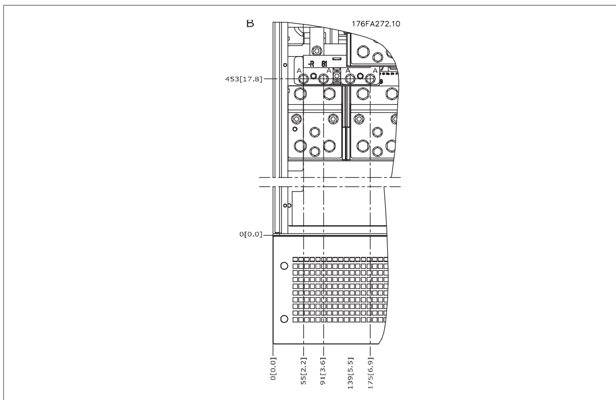
Рисунок 6.7: Расположение клемм электропитания корпусов IP21 (NEMA тип 1) и IP54 (NEMA тип 12) (фрагмент В)
