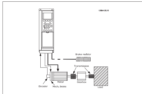
Рисунок 7.1: Базовая система регулирования скорости с обратной связью для FC 302.
