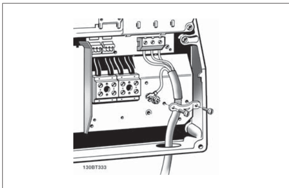
Рисунок 6.26: Подключение двигателей к преобразователям в корпусах V1 и V2 (IP 21/ NEMA, тип 1, IP 55/ NEMA, тип 12 и IP66/ NEMA, тип 4X).
