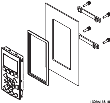
Рисунок 8.4: Монтажный комплект для LCP, включающий графическую панель LCP, крепеж, кабель (3 м) и прокладку
