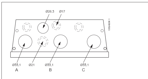
Рисунок 6.31: Отверстия ввода кабелей для корпуса V1. Предлагаемое использование отверстий является рекомендуемым, но не единственно возможным решением.
