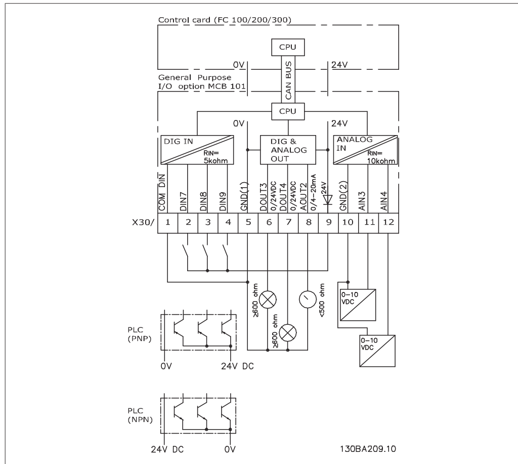
Рисунок 3.10: Принципиальная схема
