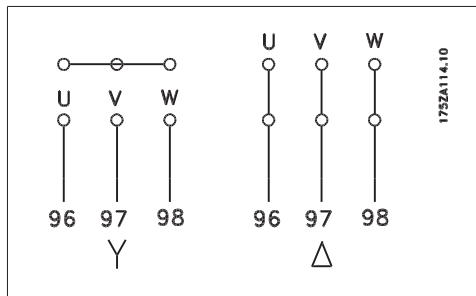
Рисунок 5.11: Подключение двигателя в случае корпусов С1 и С2.
